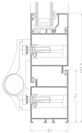
ŘEZ DVEŘE
